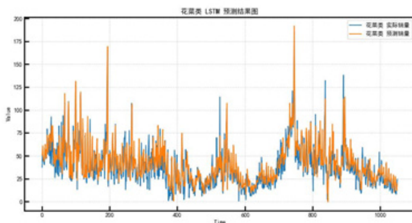
图 22 花菜类 LSTM
