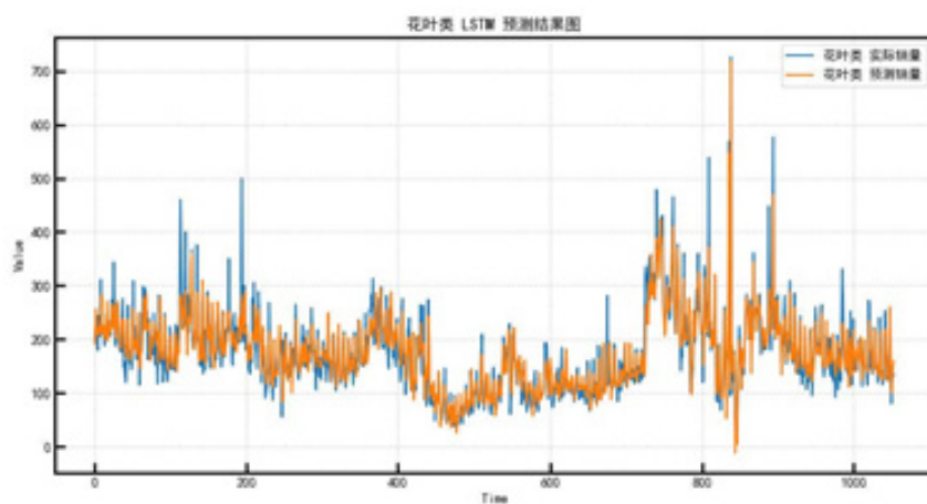
图 21 花叶类 LSTM
