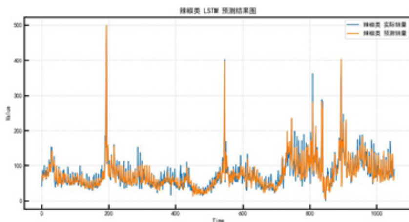
图 25 辣椒类 LSTM
