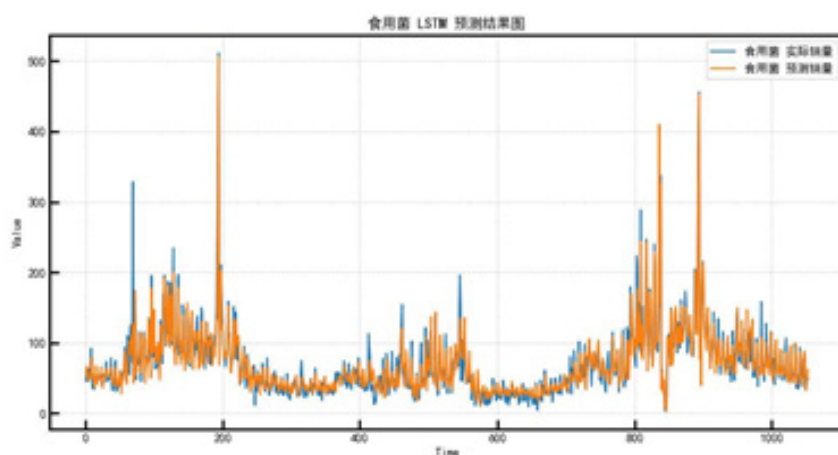
图 26 食用菌 LSTM
