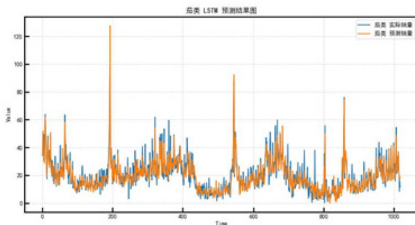
图 24 茄类 LSTM
